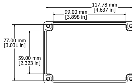
LID - INSIDE
